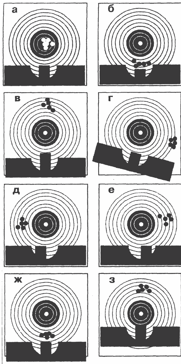
Рисунок 11. Типичные ошибки прицеливания с открытым прицелом: а – правильное прицеливание; б – «мелкая» мушка – пробоины ниже цели; в – «крупная» мушка – пробоины выше цели; г – оружие «свалено» вправо – пробоины правее и ниже; д – мушка левее центра прорези прицела – пробоины левее цели; е – мушка правее центра прорези прицела – пробоины правее цели; ж – большой просвет – пробоины ниже цели; з – мушка в яблочке – пробоины выше цели
