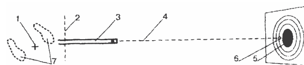
Рисунок 6. Схема стрельбы стоя. Вид сверху: 1 – проекция центра тяжести стрелка; 2 – линия огня; 3 – ствол винтовки; 4 – линия прицеливания; 5 – яблочко мишени; 6 – точка прицеливания; 7 – следы ног
