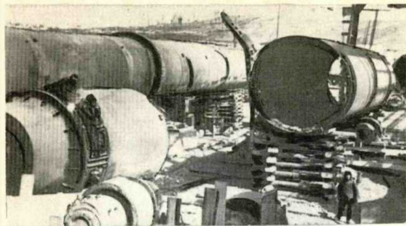
Строится Теплоозерский цементный завод. Идет монтаж вращающихся печей. 1957 г.
